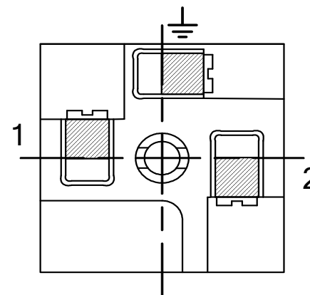
Расположение контактов на розетке разъема со стороны винтового закрепления проводников (Разъем в соответствии DIN 43650C серии GDM с 3 контактами).
