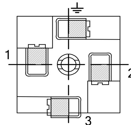
Расположение контактов на розетке разъема со стороны винтового закрепления проводников (Разъем в соответствии DIN 43650C серии GDM с 4 контактами).
