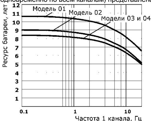
Рис. 1.1 – Ресурс батареи
