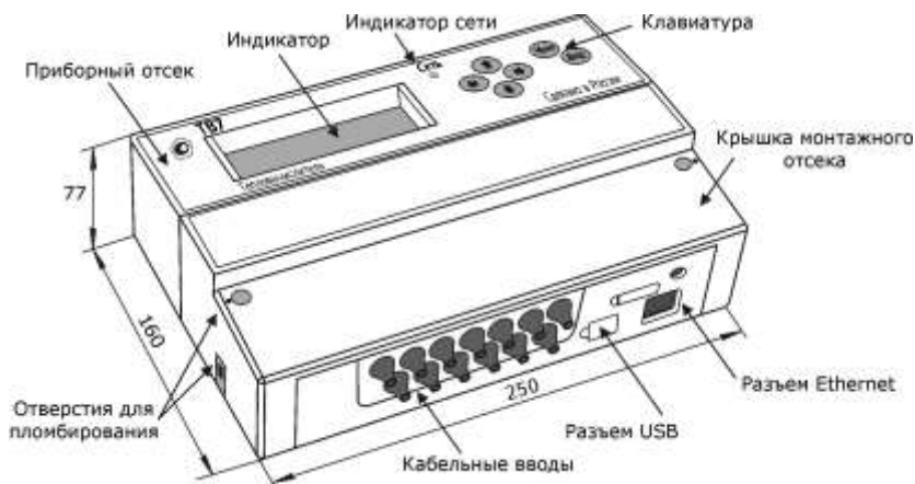
Рис. 2.1 – Внешний вид ТВ7
