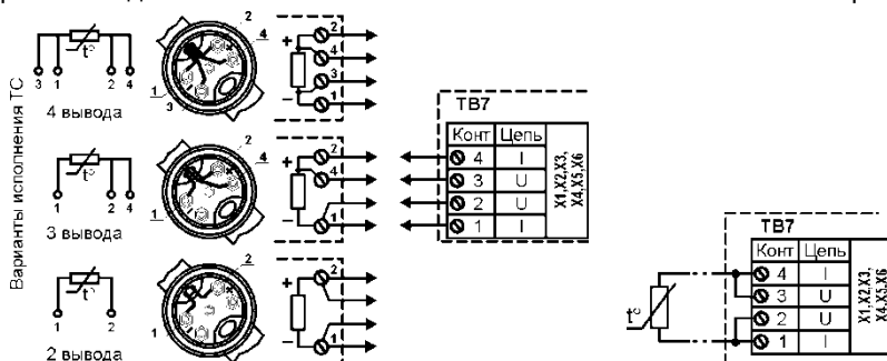
а) Подключение ТС по 4-проводной схеме б) Подключение 2-х проводных ТС
