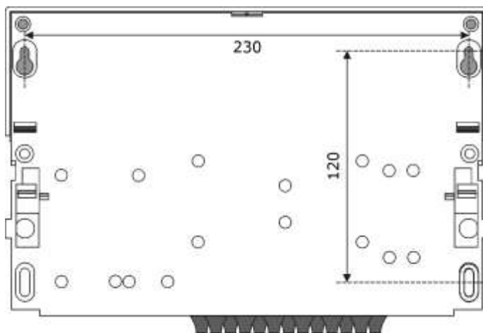
Рис. 4.1 – Схема крепления корпуса ТВ7
