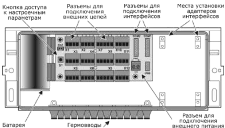
Рис. 2.2 – Вид на монтажный отсек при снятой крышке
