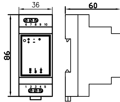
Рис. 1 - Габаритный чертеж
