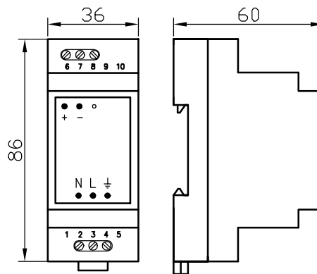
Рис. 1 - Габаритный чертёж
