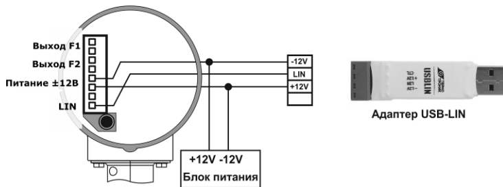
Рис. 7 – Схема подключения адаптера USB
