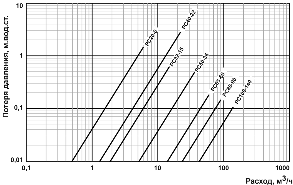
Потери давления на Питерфлоу РС с L-каналом
