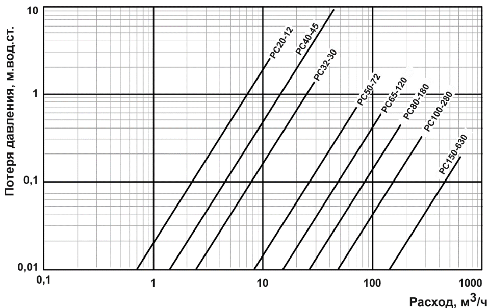
Потери давления на Питерфлоу РС с полнопроходным каналом
