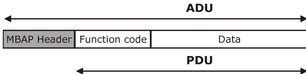
Рисунок 5: ADU для «Modbus TCP»
