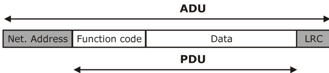
Рисунок 4: ADU для «Modbus ASCII»
