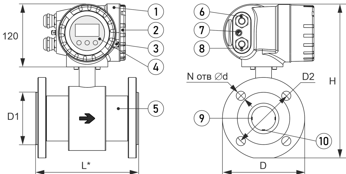
Рисунок А.1 Внешний вид и габаритные характеристики расходомеров единого исполнения
