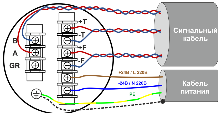
Рисунок 3.17 Подключение внешних соединений
