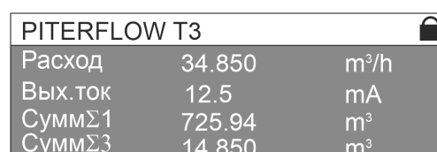
Рисунок 2.12 Главный экран в режиме индикации четырех параметров
