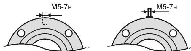
Рисунок 3.2 Доработка фланцев
