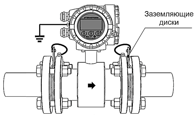
Рисунок 3.16 Заземление расходомера на пластиковых трубах с заземляющими дисками
