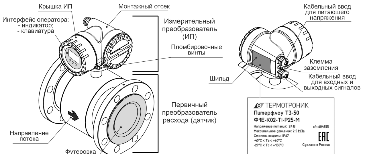
Рисунок 2.2 Внешний вид расходомера единого исполнения
