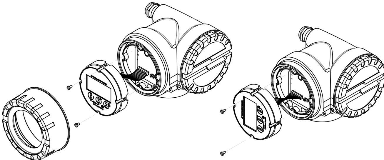
Рисунок 3.3 Поворот индикатора расходомера
