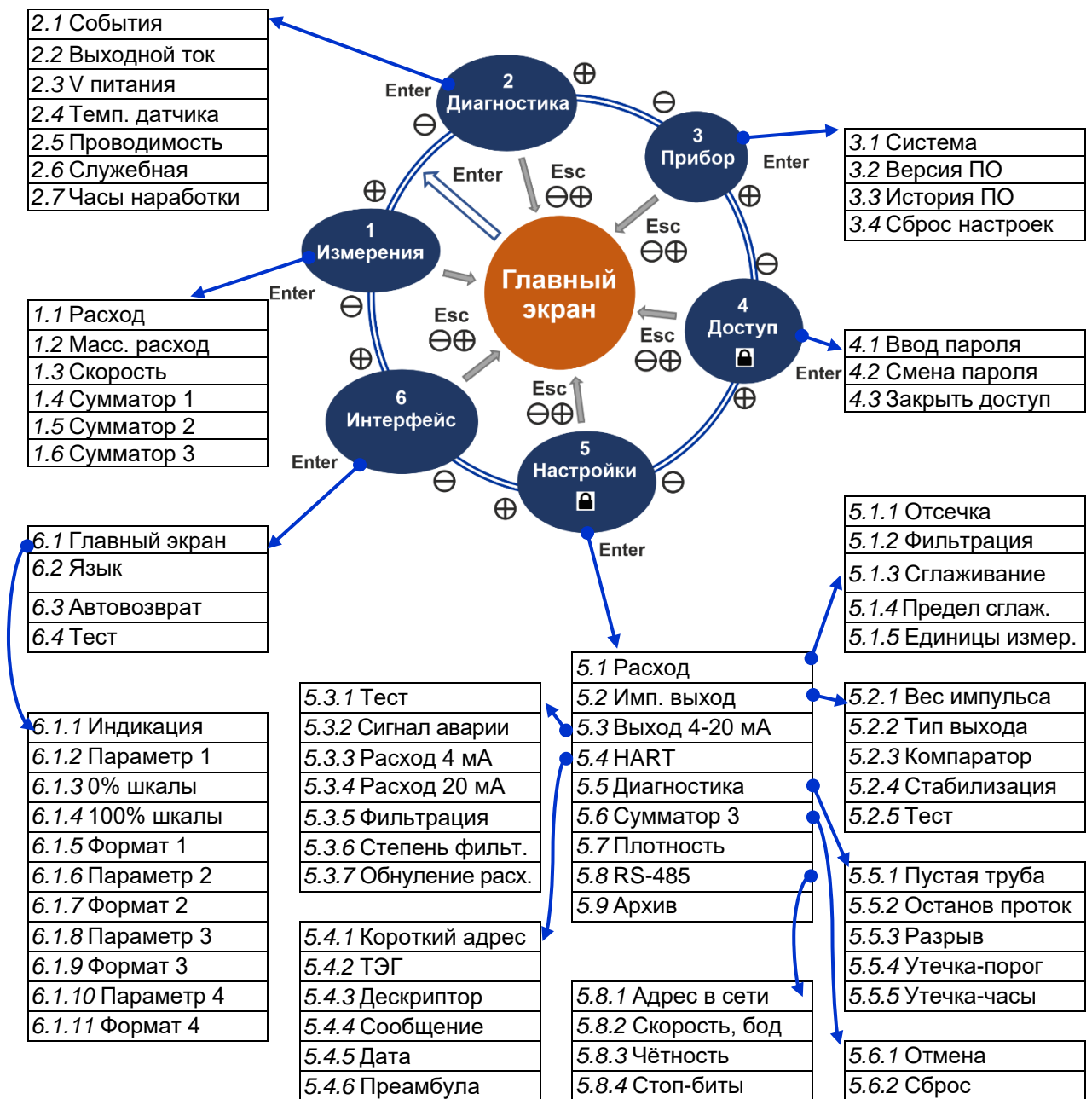
Рисунок 2.18. Общая структура меню расходомера
