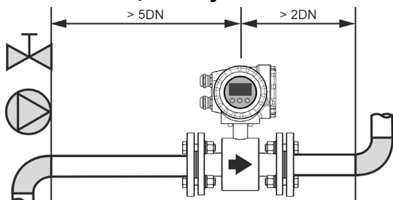
Рисунок 3.4 Длины прямых участков
