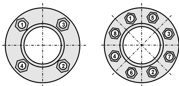
Рисунок 3.14 Порядок затяжки гаек
