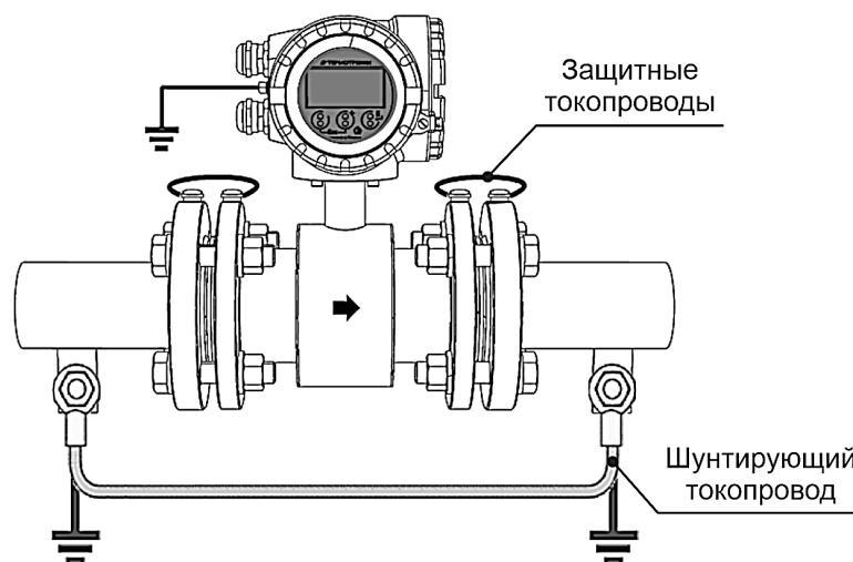
Рисунок 3.15 Выравнивание потенциалов в металлических трубах
