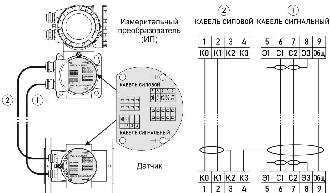
Рисунок 3.17 Схема подключения датчика к ИП раздельного исполнения
