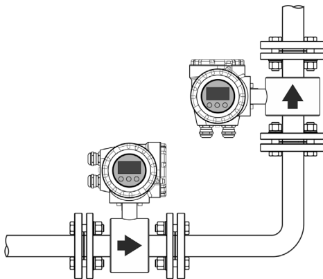
Рисунок 3.7 Рекомендуемые варианты установки
