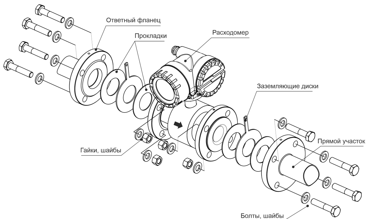
Рисунок 3.13 Установка расходомера
