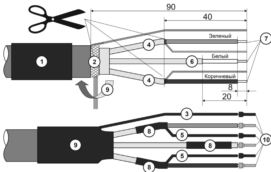
Рисунок 3.18 Порядок действий при подготовке сигнального кабеля
