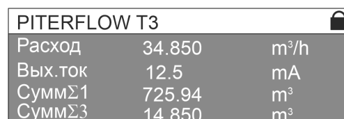
Рисунок 2.14 Главный экран в режиме индикации четырех параметров
