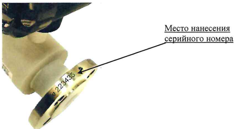
Рисунок 7 – Место нанесения заводского номера на расходомер-счётчик Питерфлю Т модификации 1
