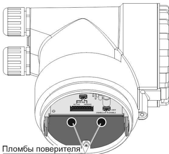
Рисунок 2.24 Пломбирование доступа к изменению метрологически значимых параметров
