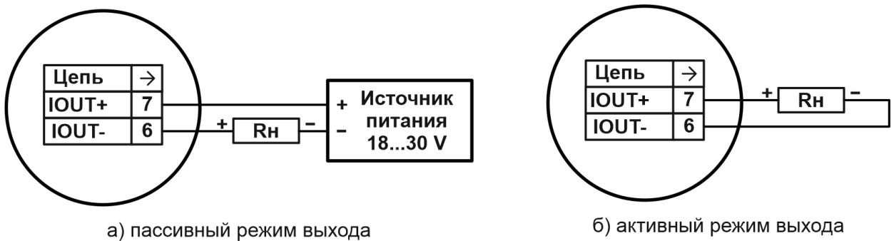
Рисунок 2.10 Схема подключения токового выхода
