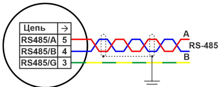
Рисунок 2.11 Подключение интерфейса RS-485
