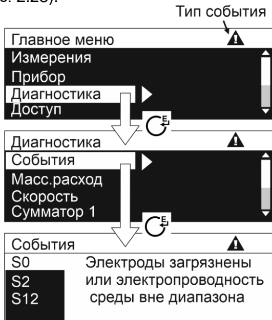
Рисунок 2.23. Просмотр кодов событий
