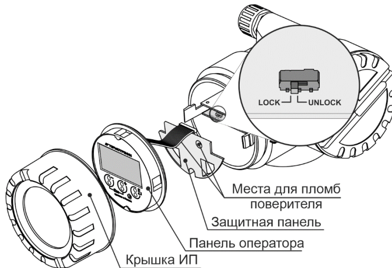
Рисунок 2.5 Переключатель режимов работы
