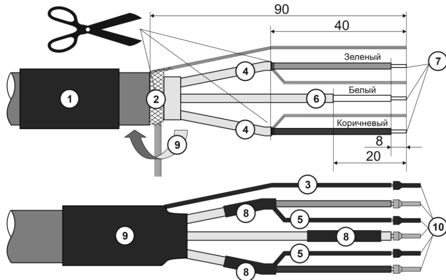
Рисунок 3.23 Порядок действий при подготовке сигнального кабеля
