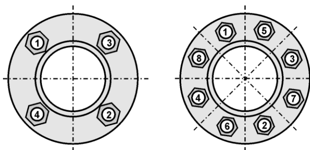
Рисунок 3.15 Порядок затяжки гаек
