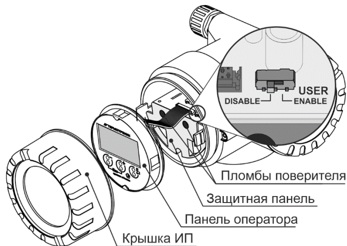
Рисунок 2.6 Расположение переключателя доступа
