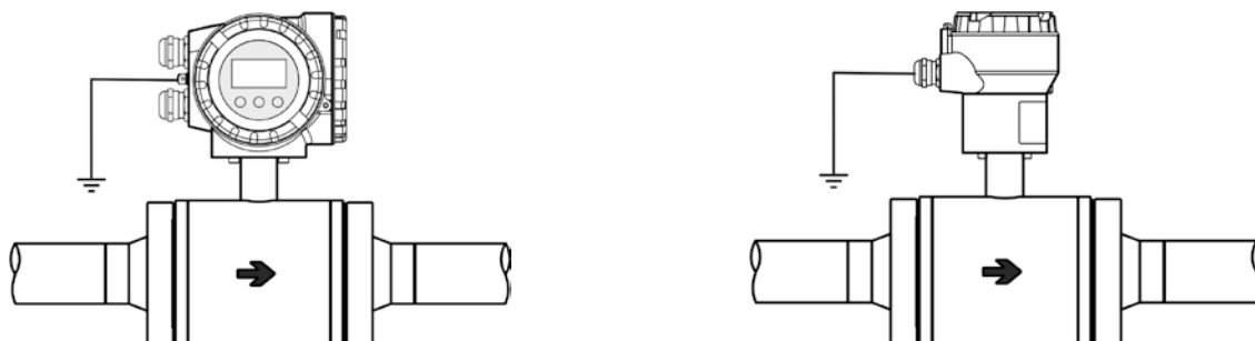
Рисунок 3.17 Защитное заземление
