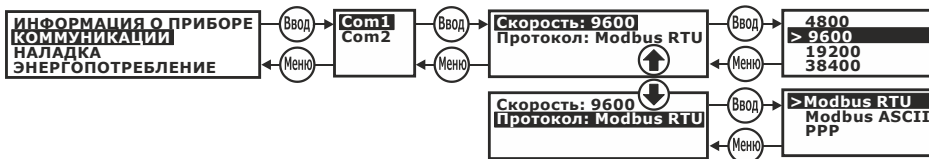
Рис. 3.13 – Настройка Com-портов
