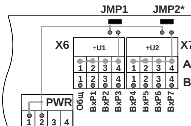
Рис. 4.5 – Организация питания датчиков давления
