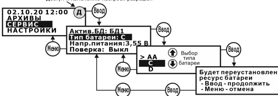
Рис.И.2 – Порядок установки/выбора типа батареи
