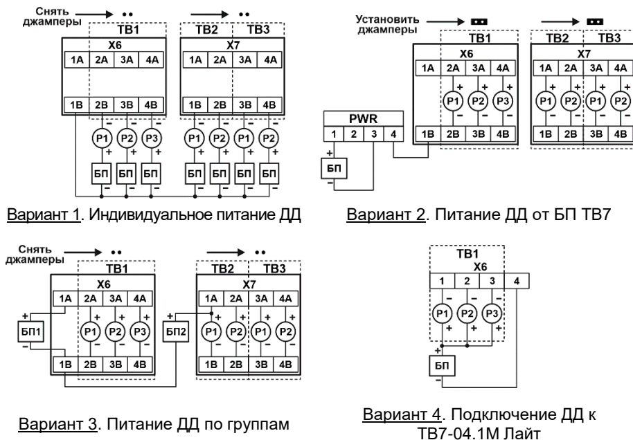
Рис. 4.6 – Варианты подключения датчиков давления к ТВ7
