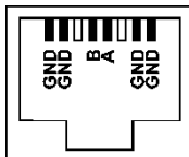
Рис. Ж.2 Цоколевка выходов разъема RJ45
