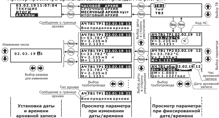
Рис. 3.7 – Примеры вывода на индикатор архивных величин
