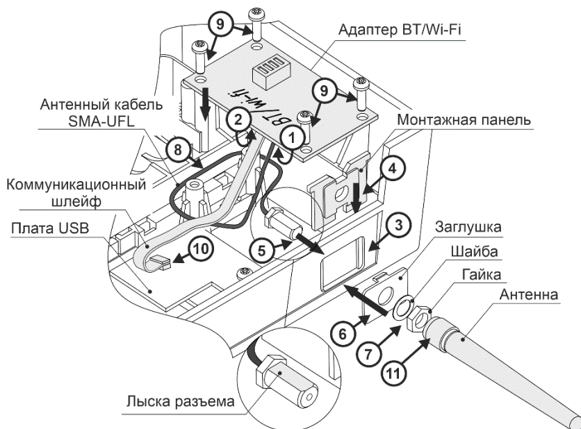
Рис. 3.2 Порядок установки адаптера
