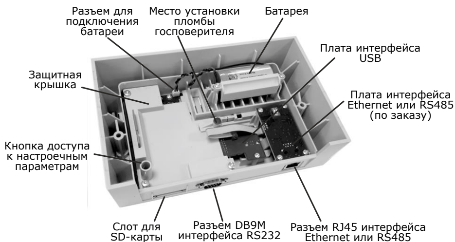
Рис. 2.2 – Вид снизу на приборный отсек TB7
