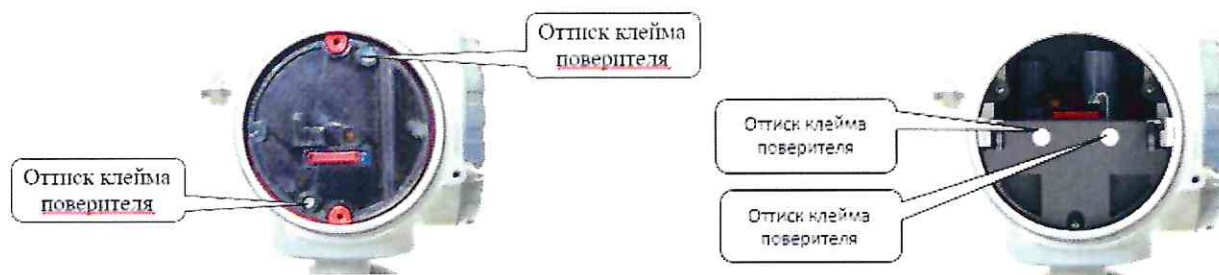
Рисунок 4 – Места нанесения знака поверки на ИП расходомера-счётчика Питерфлоу Т модификации 3
