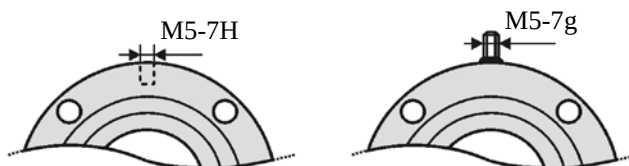
Рис. 6.11 Доработка фланцев
