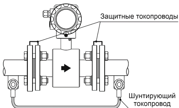
Рис. 6.15 Подключение защитных и шунтирующего токопроводов
