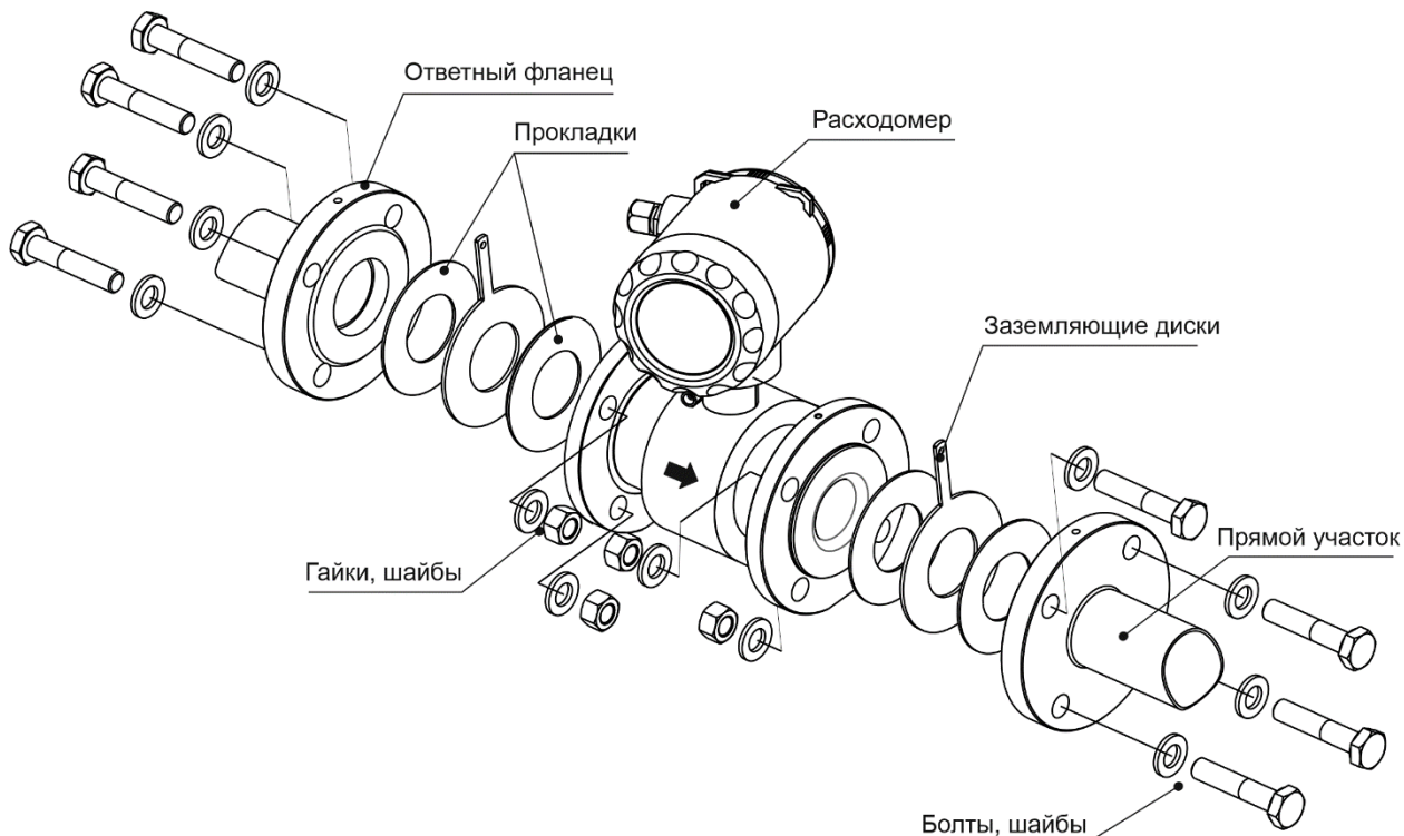
Рис. 6.10 Установка расходомера
