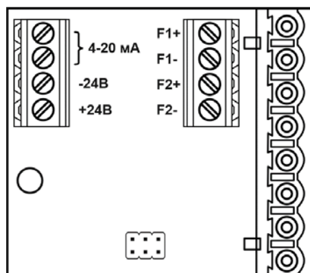
Рис. В.1 Адаптер PCA
